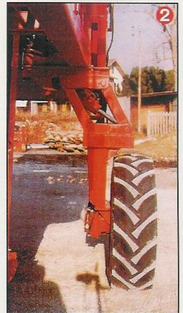
2 Carreggiata larga in fase di lavoro (m. 3,44) Working wheel tread (m. 3,44)
